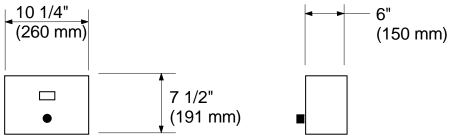
INDICATOR BOX
