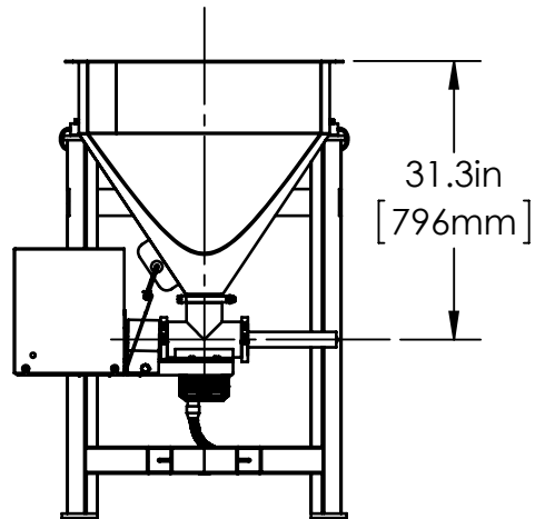
SECTION A-A SCALE 1:24
